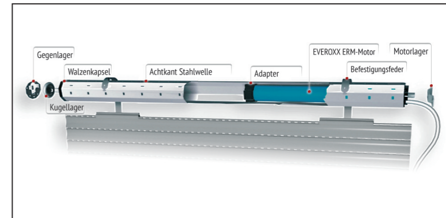
Abb.: Montagebeispiel
