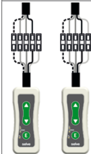
4 fils
