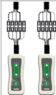
4-adrig 5-adrig
