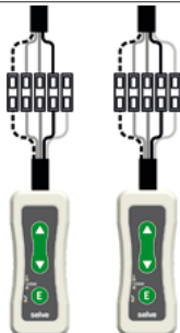
4 wire
